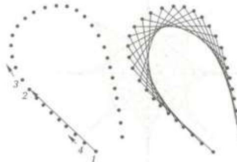
Рис. 43. Заполнение окружности со смещенным центром
